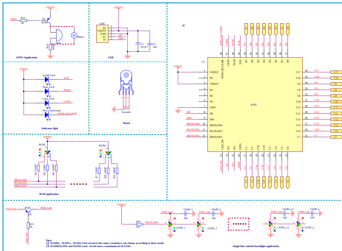
图 7-1 典型应用电路
