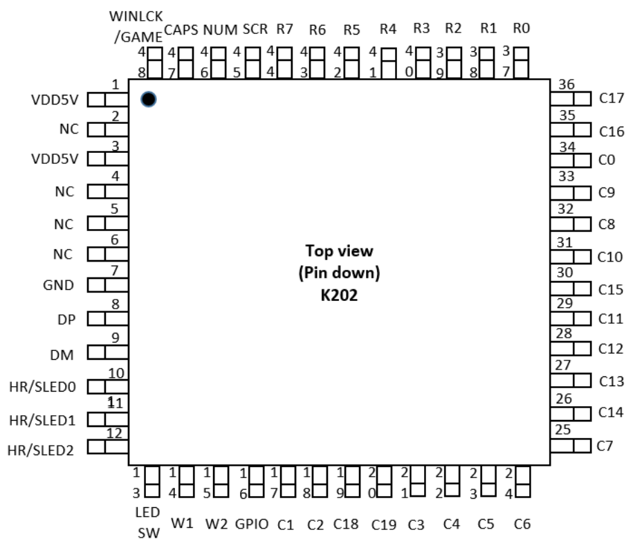
图 8-1. Pin 定位
