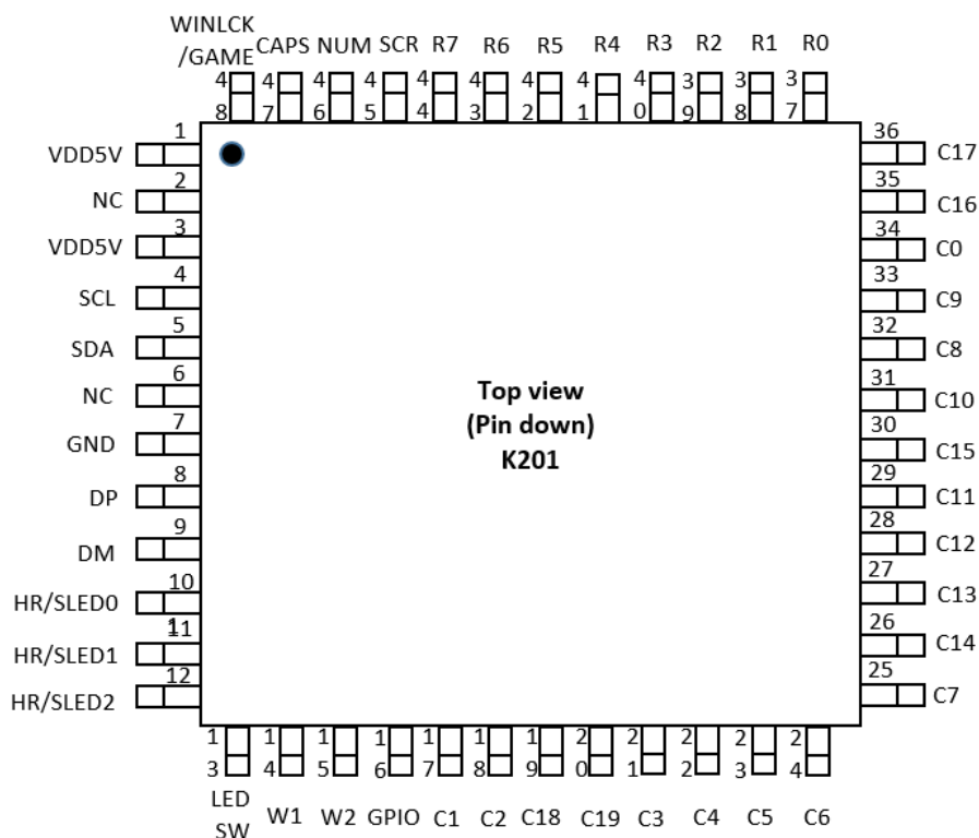
图 4-1. Pin 排列
