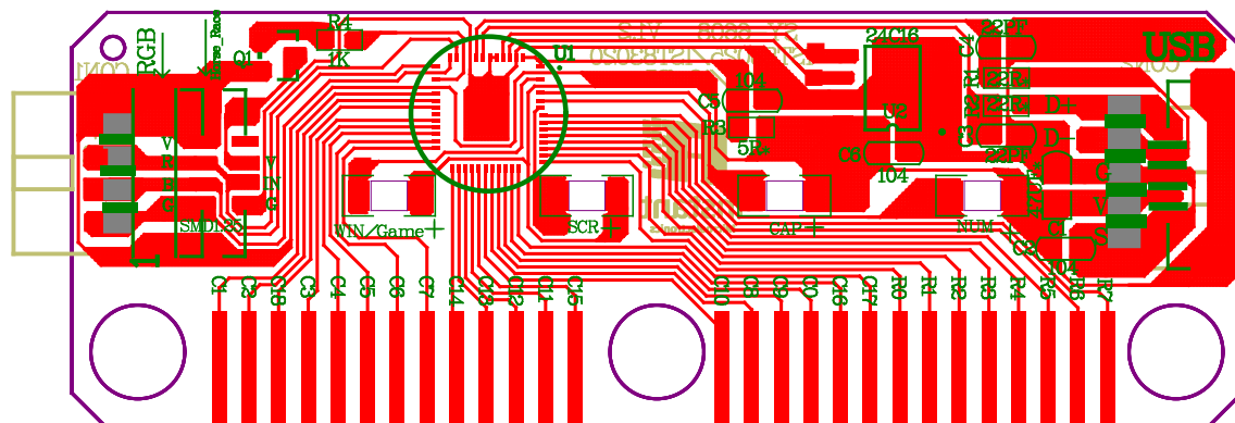
图 9-1 典型应用 PCB
