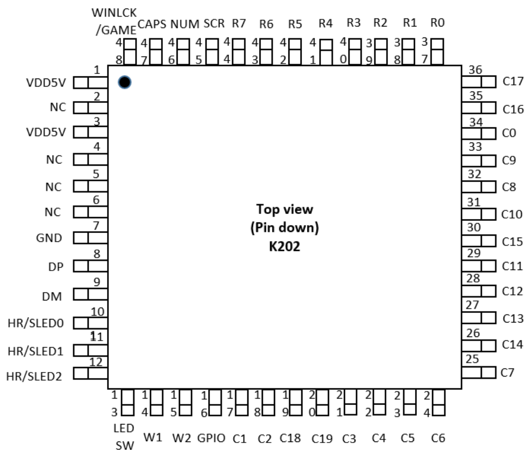
图 8-1. Pin 定位
