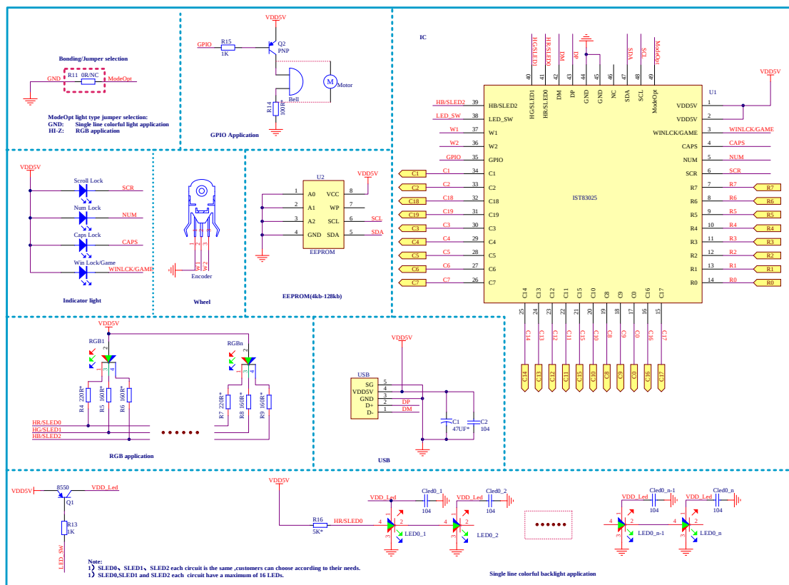
图 7-1 典型应用电路
