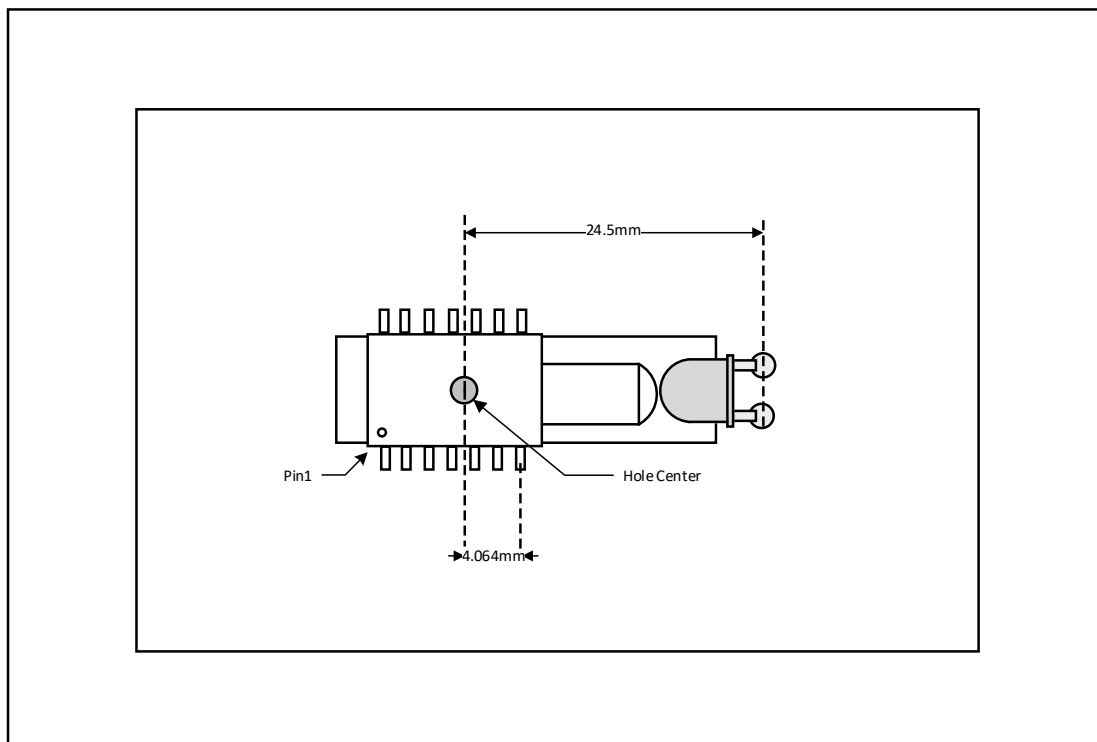
图 5.2D 装配俯视图
