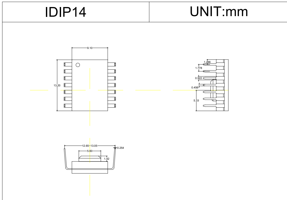
图 4. 封装外观图
