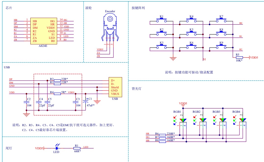
图 3. 应用电路图
