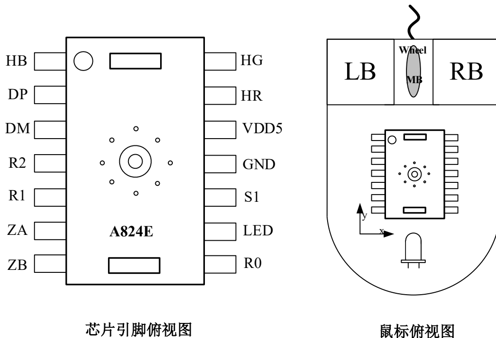
图 1. 引脚排列图
