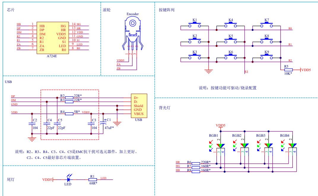
图 3. 应用电路图
