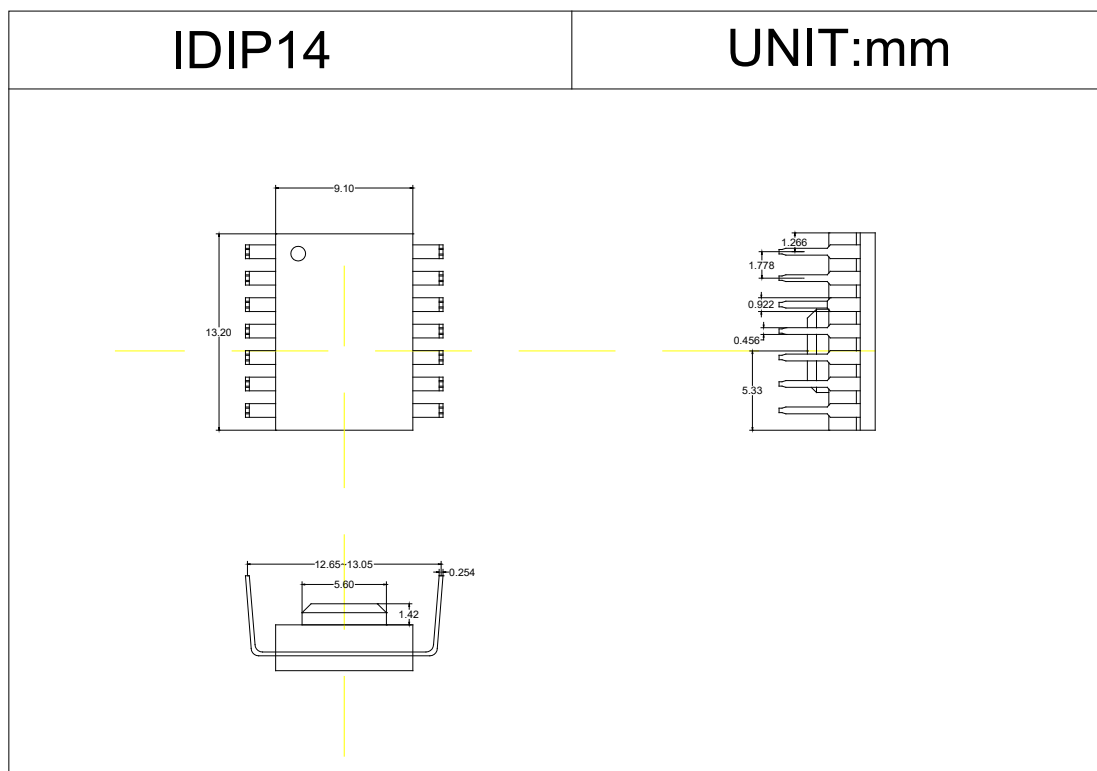
图 4. 封装外观图
