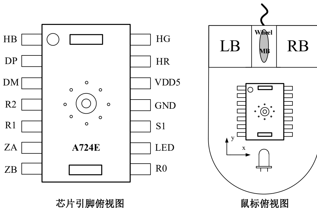
图 1. 引脚排列图
