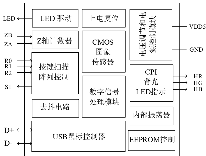
图 2. 模块框图
