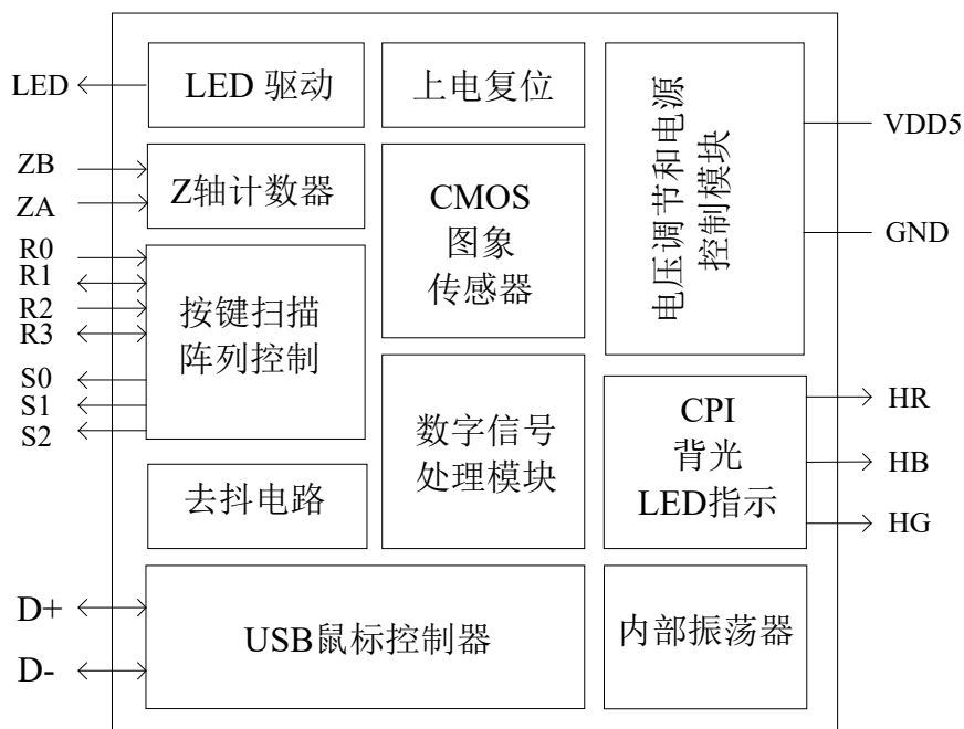
图 2. 模块框图
