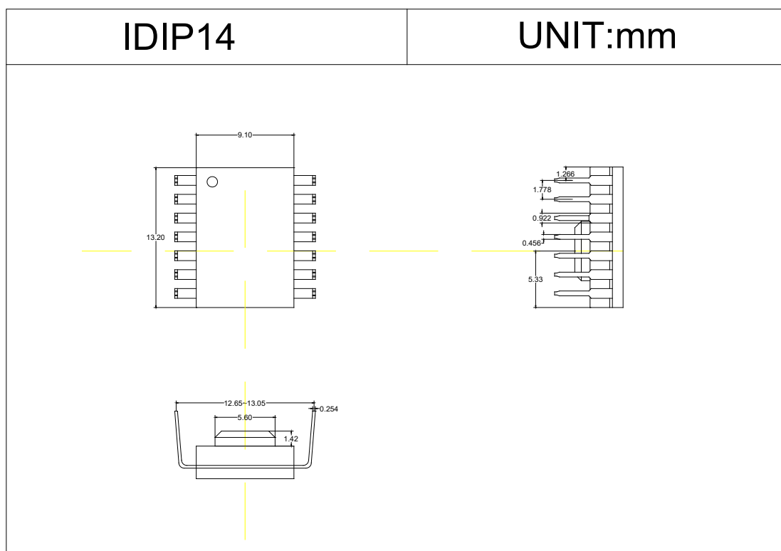
图 4. 封装外观图
