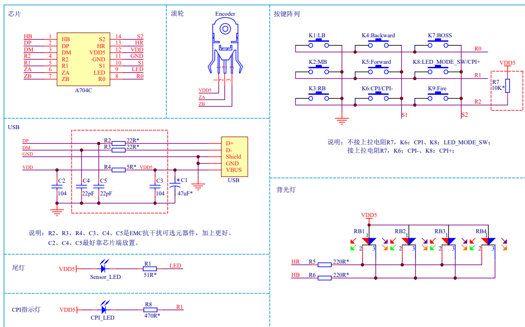
图 3. 应用电路图
