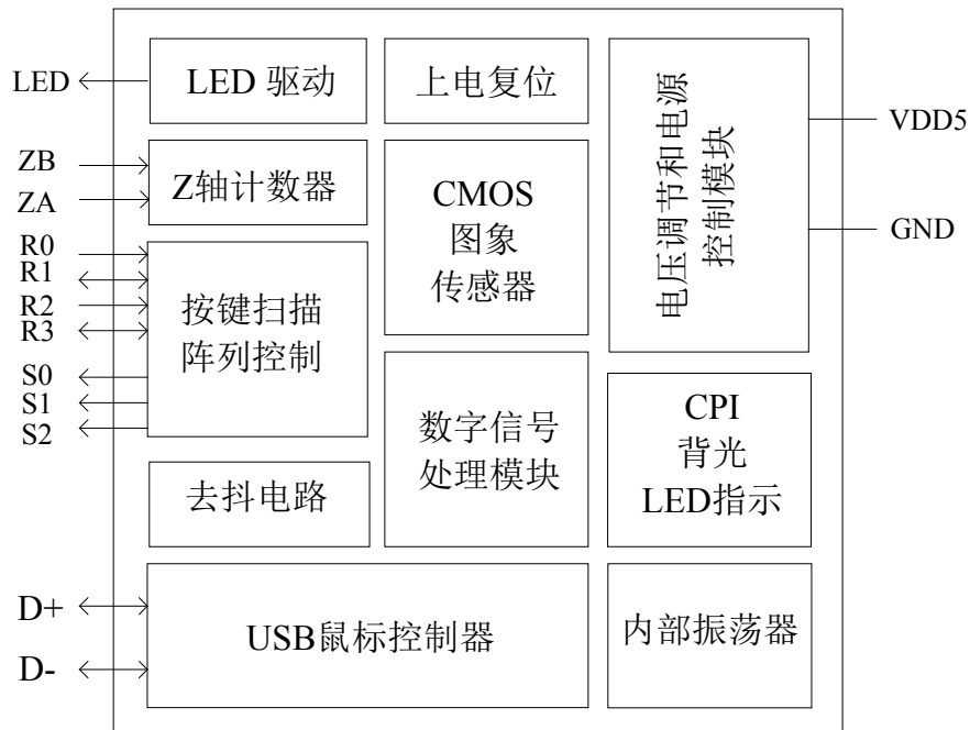
图 2. 模块框图
