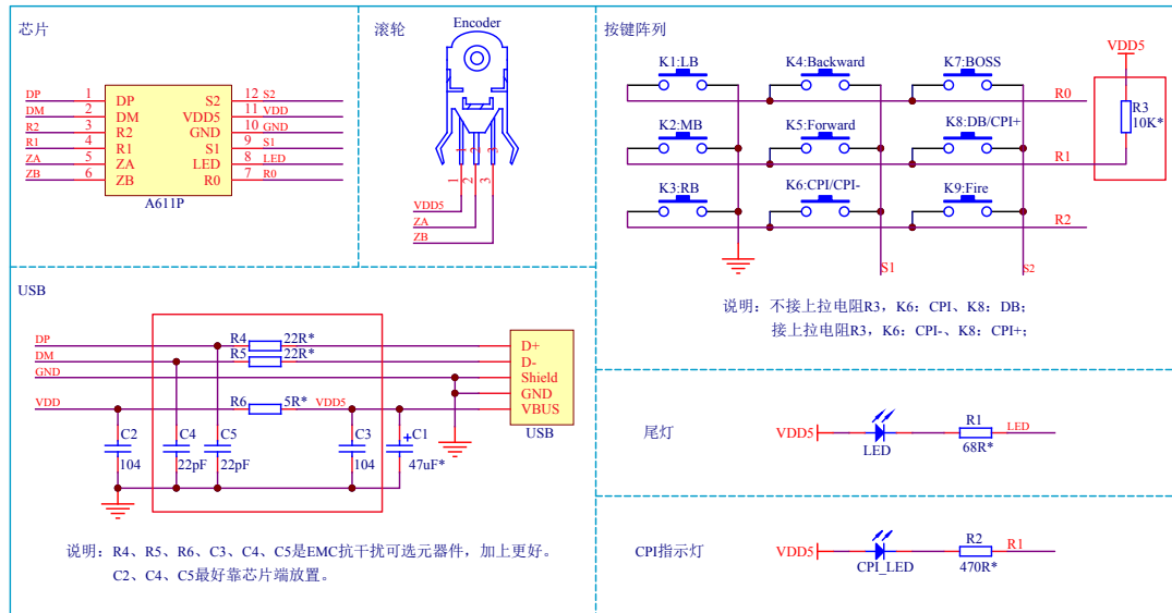
图 3. 应用电路图
