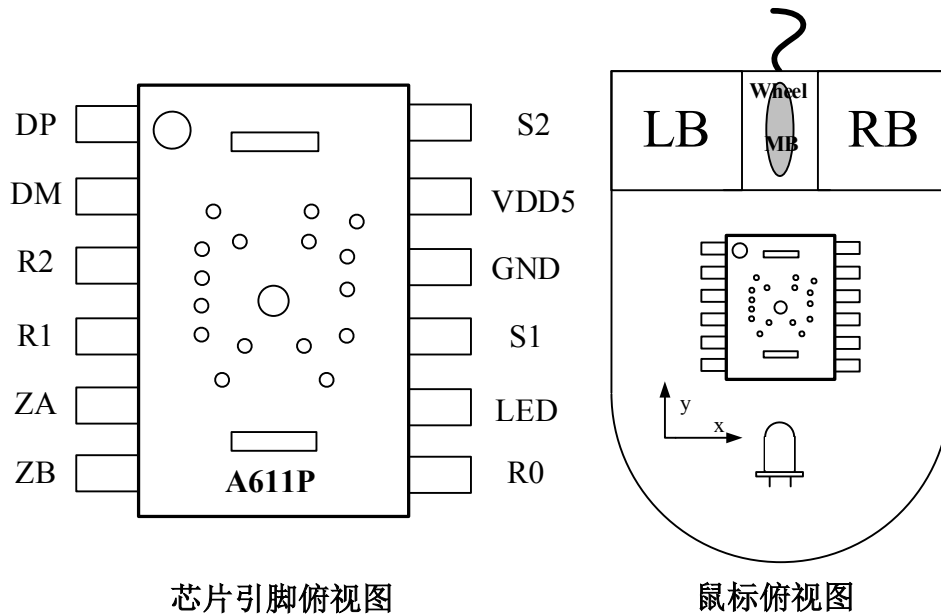
图 1. 引脚排列图
