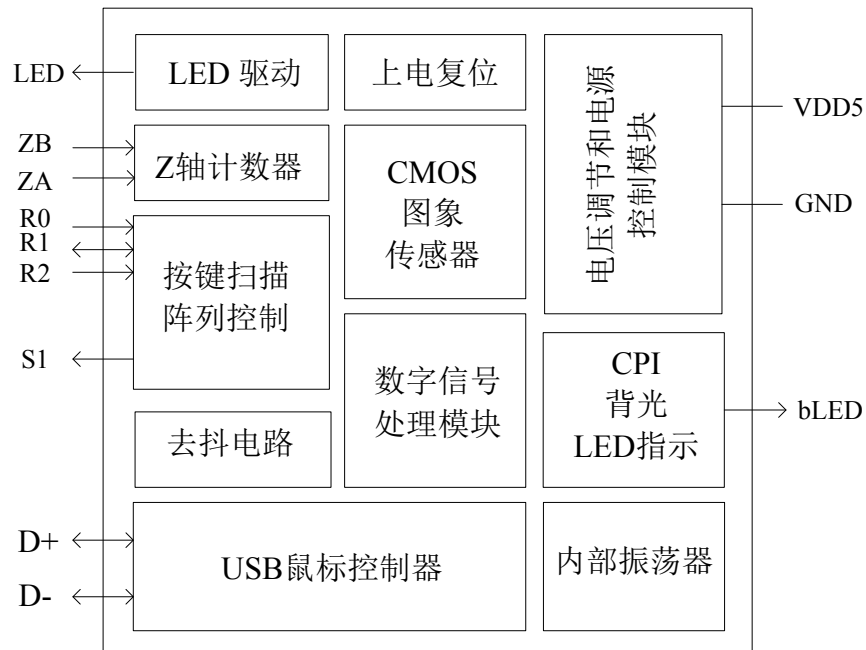
图 2. 模块框图
