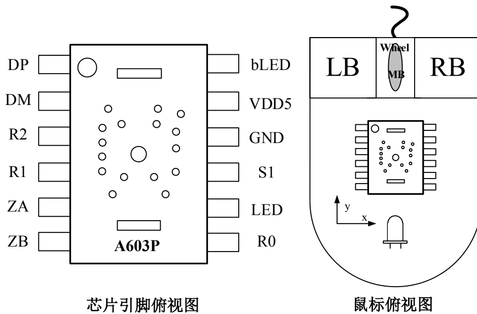
图 1. 引脚排列图
