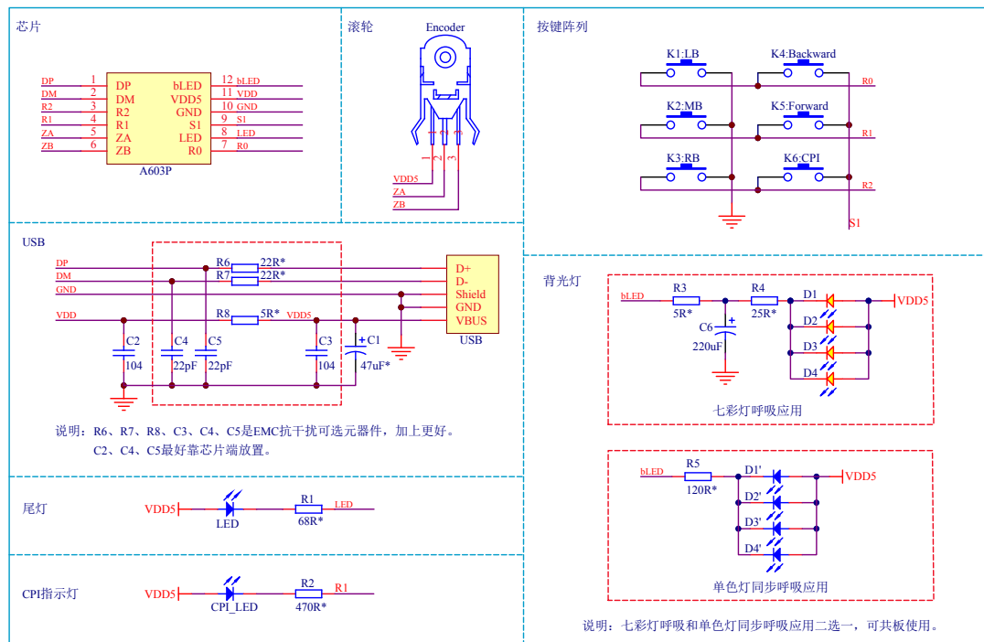
图 3. 应用电路图
