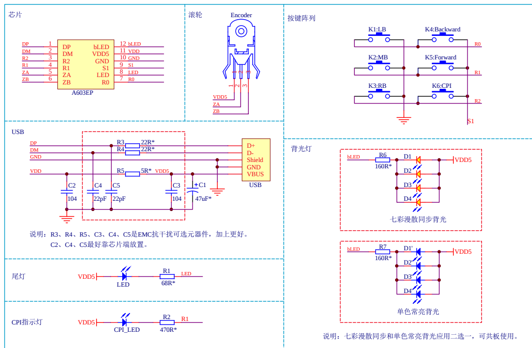
图 3. 应用电路图
