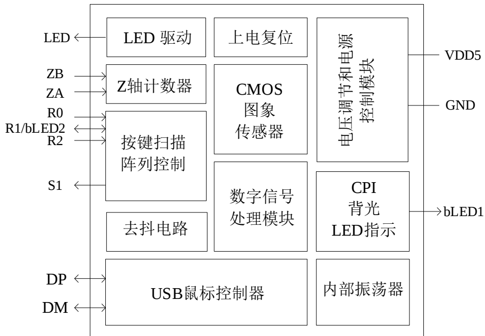
图 2. 模块框图
