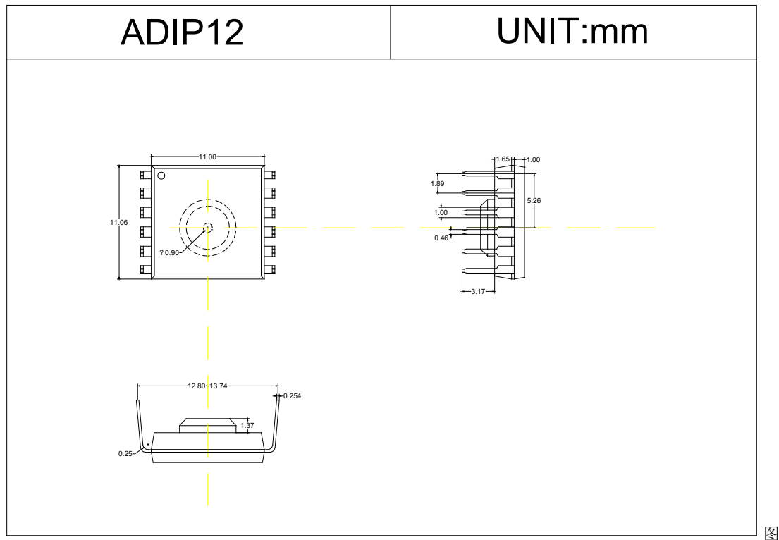
4. 封装外观图
