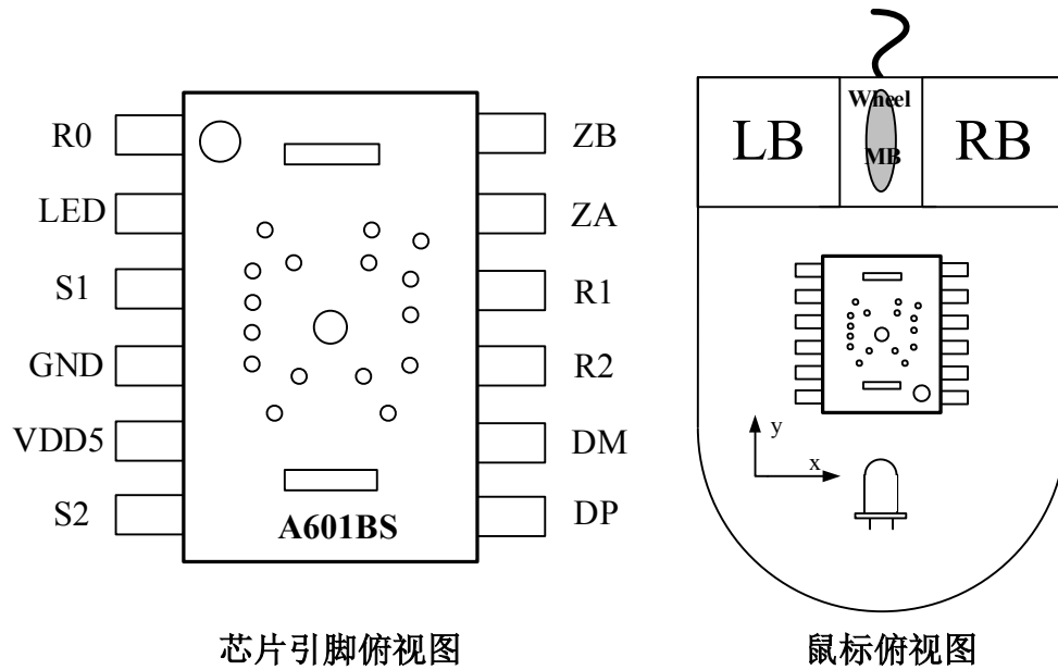
图 1. 引脚排列图
